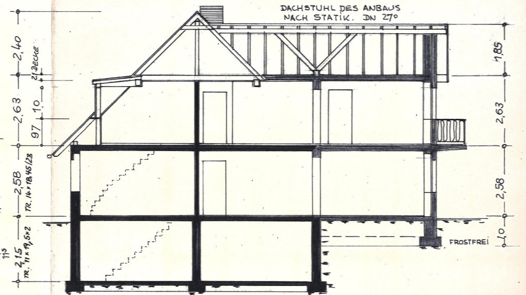
SCHNITT A - D
